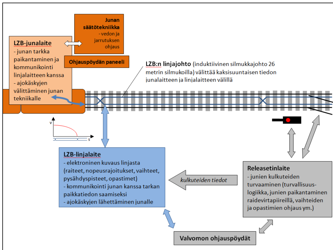
Kuva 2. Koeradon LZB-kulunvalvonnan perusperiaate. Tiedot Siemens (1973) ja Metrotoimisto (1974b).
