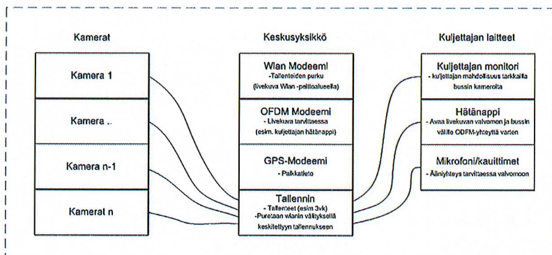
Kuva 6 Turvakamerajärjestelmän lohkokaavio (yleinen esitys).
